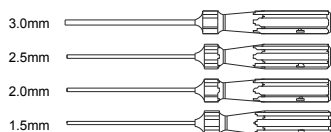
Sechskant-Schraubendreher
